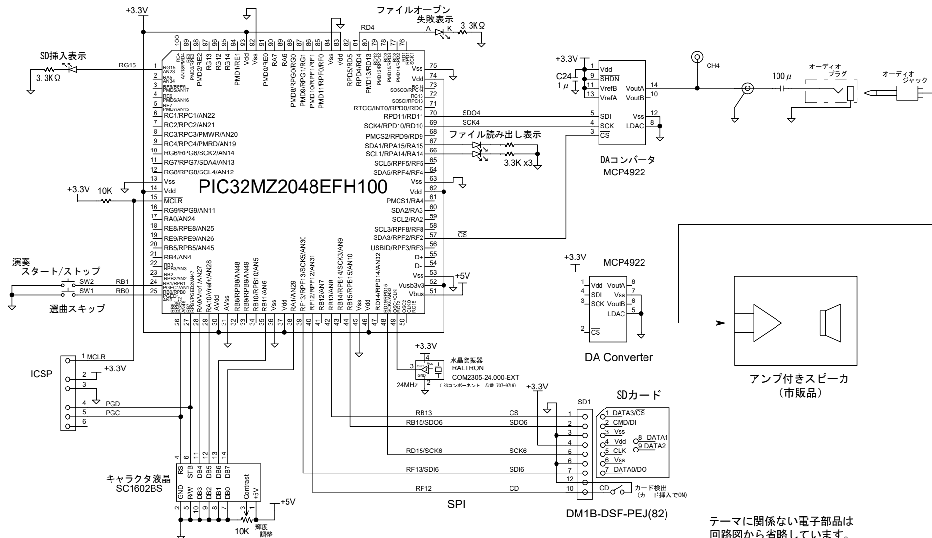
PIC32MZ DMA式 WAV プレーヤー 電気回路図
